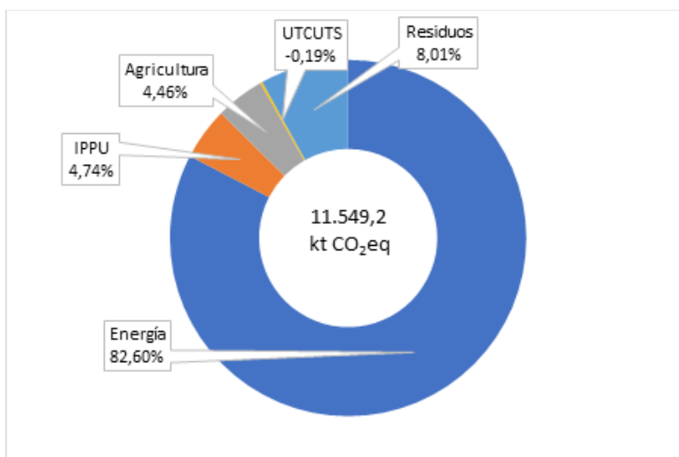
Figura 14. Aporte porcentual de sectores a emisiones de la Región del Biobío. Año 2020. Fuente: MMA
