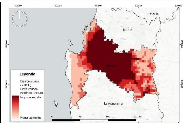
Proyección de días calurosos (>30°) en la Región del Biobío. Valor mínimo: 0 días, valor máximo: 23,6 días. F
