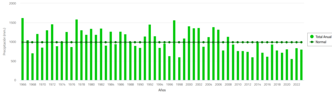
Figura 7. Precipitación Histórica Anual entre 1966 y 2023 de la Estación Carriel Sur, Concepción (código 360019). Fuente: Servicios Climáticos DMC.
