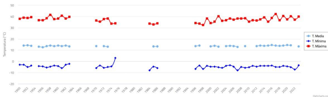
Figura 6. Temperatura histórica entre 1950 y 2023 de la Estación María Dolores, Los Ángeles (código 370033 7 ). Fuente: Servicios Climáticos DMC.
