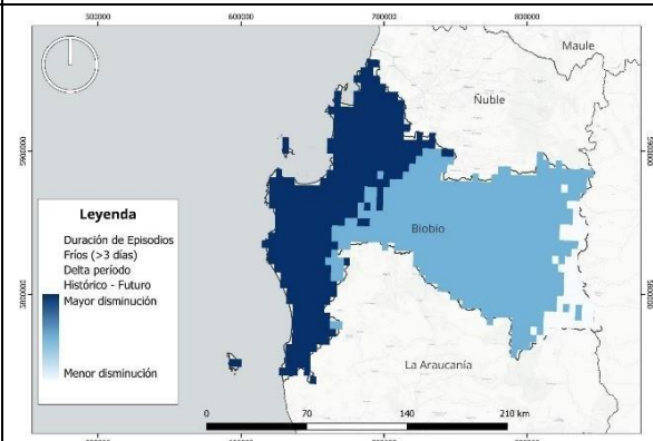
Proyección de Duración de Episodios Fríos (>3 días) en la Región del Biobío. Valor mínima disminución: -2,8 días, valor máxima disminución: -5,0 días.
