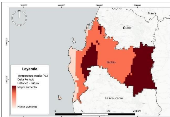
Proyección en la temperatura media anual en la Región del Biobío. Valor mínimo: 0,6°C, valor máximo: 1,5 °C.
